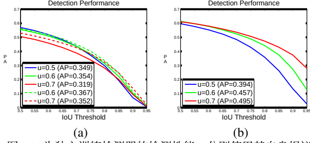
图5. (a)为独立训练检测器的检测性能，分别使用其自身提议（实线曲线）或级联R-CNN阶段提议（虚线曲线），(b)为在提议集中加入真实标注后的检测性能。
